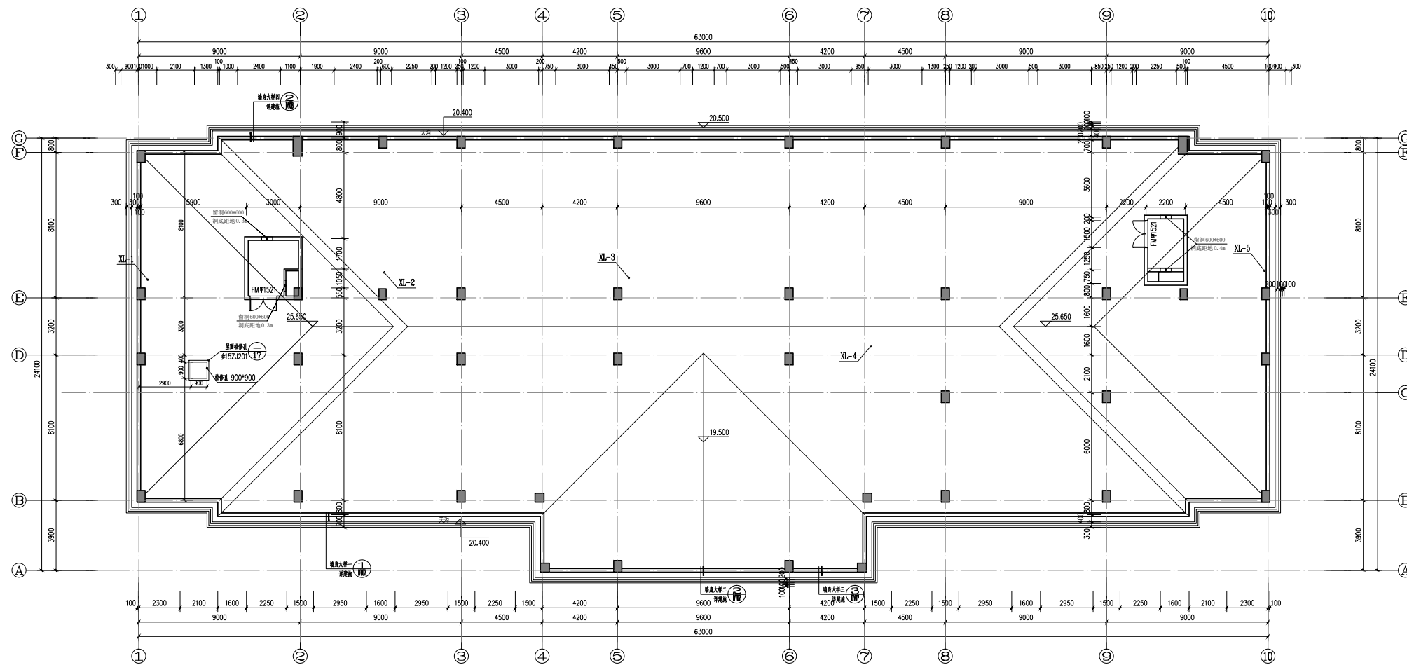
D-2#楼(党校教学综合楼) 闷顶层平面图 (变更前) 1:100
