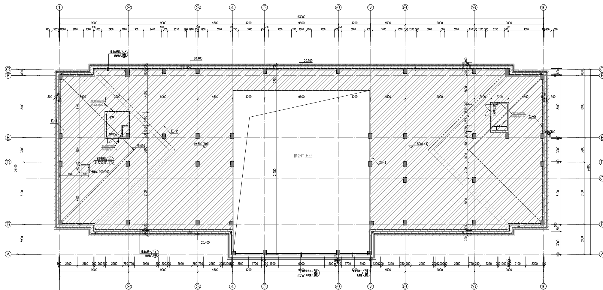
D-2#楼(党校教学综合楼) 闷顶层平面图 (变更后) 1:100
