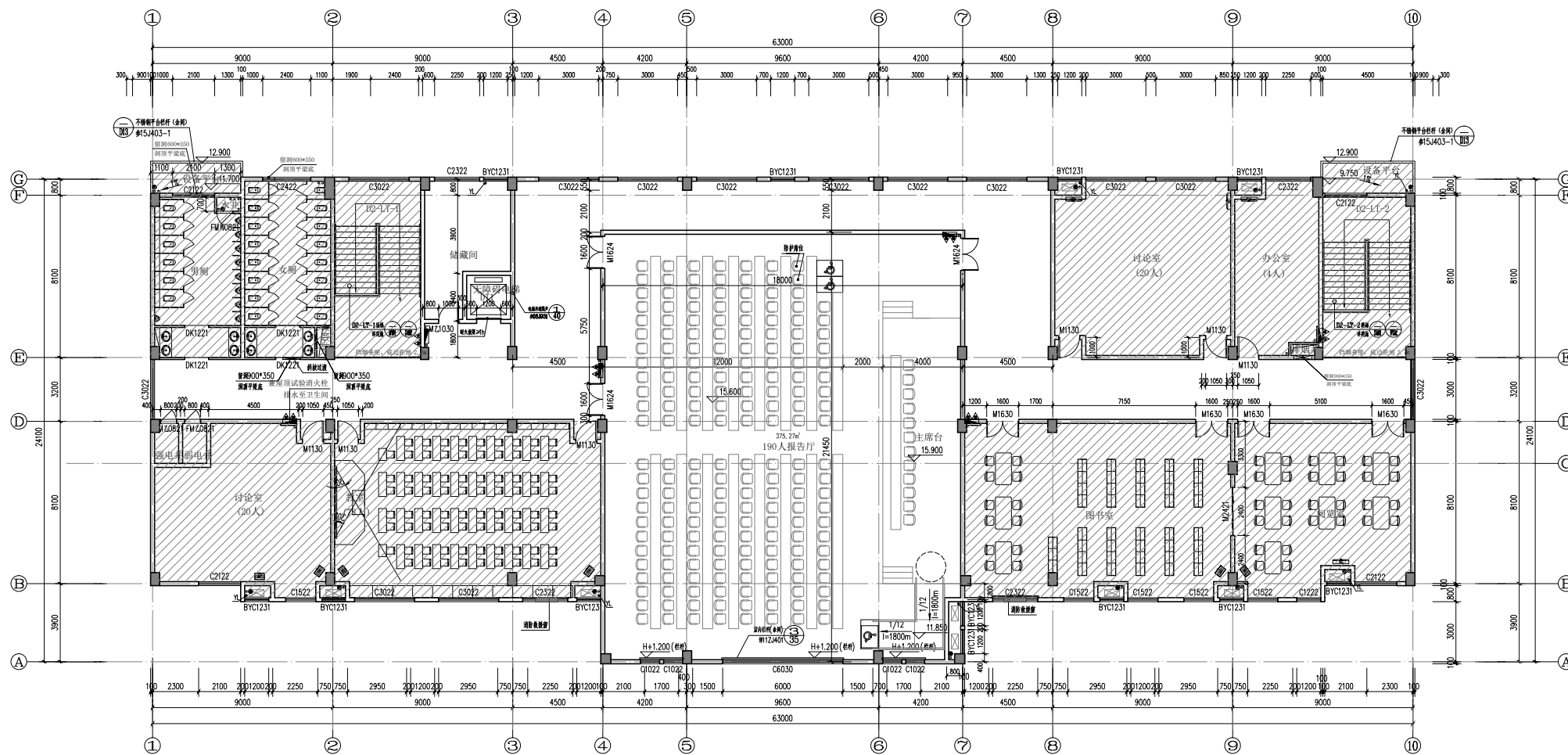
D-2#楼(党校教学综合楼) 五层平面图(变更后) 1:100
