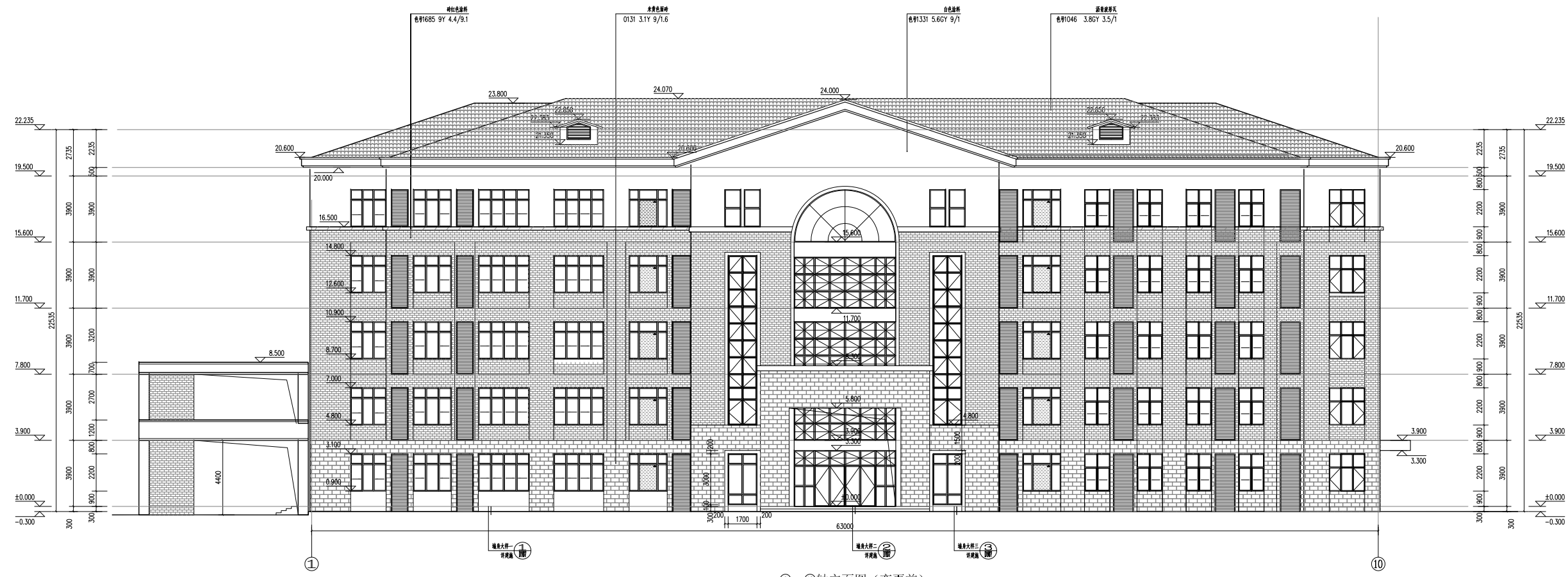
①-⑩轴立面图 (变更前) 1:100
