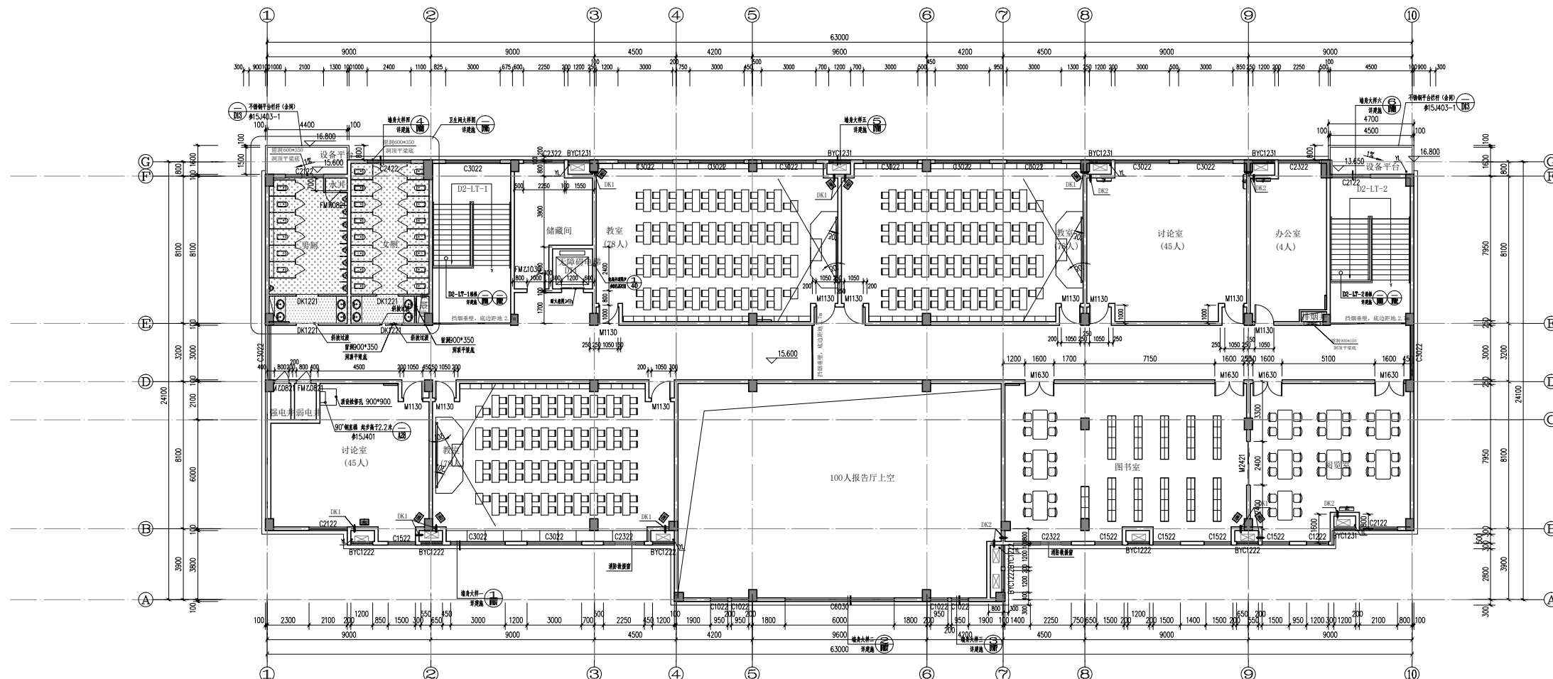
D-2#楼(党校教学综合楼) 五层平面图(变更前) 1:100
